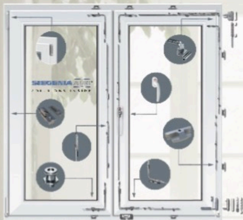
Esquema de Herraje Gama Classic
